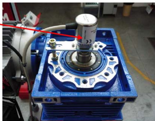
COLONNA CON DETTAGLIO ENCODER ASSOLUTO E SCHEDA MICROPROCESSORE
